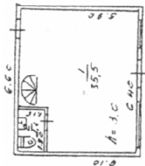
1 этаж
